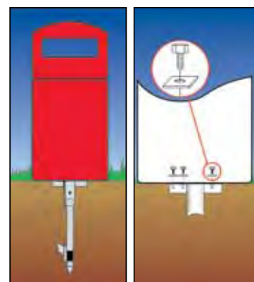
Papera instalada con el sistema de anclaje Glasdon.
